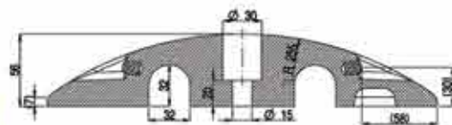
A-A SCALE 1:2
